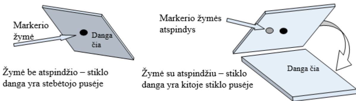
12 pav. Stiklo Stopsol dangos pusės nustatymas.
