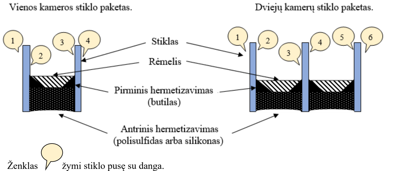
1 pav. Stiklo paketo struktūrinė diagrama.
