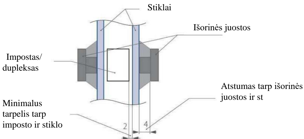
14 pav. Impostų/dupleksų pozicionavimo tikslumas stiklo paketo kameroje tarpusavyje ir stiklo paketo kraštų atžvilgiu.
