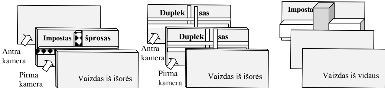
13 pav. Impostų/dupleksų sumontavimas, stiklo pakete.
