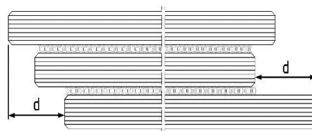
5 pav. Stiklo paketo stiklų prasikeitimas.
